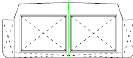
Typ G Konštrukcia nákladného tanku 2 Typ nákladného tanku 2 (aj s hladkou palubou)
