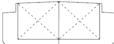
Typ N Konštrukcia nákladného tanku 2,3 a 4 Typ nákladného tanku 1 (aj s hladkou palubou) (také s hladkou palubou)
