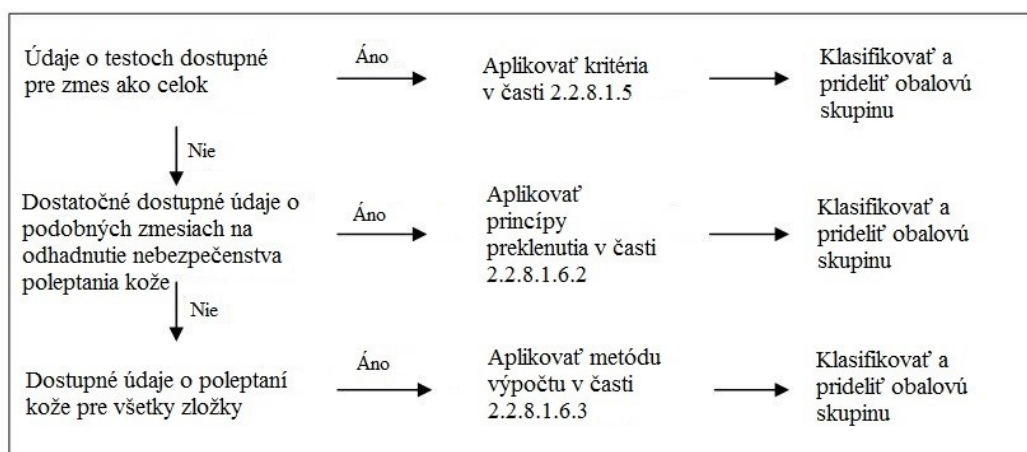
Obr. 2.2.8.1.6.1: Stupňovitý prístup ku klasifikácii a prideleniu obalovej skupiny žieravých zmesí
