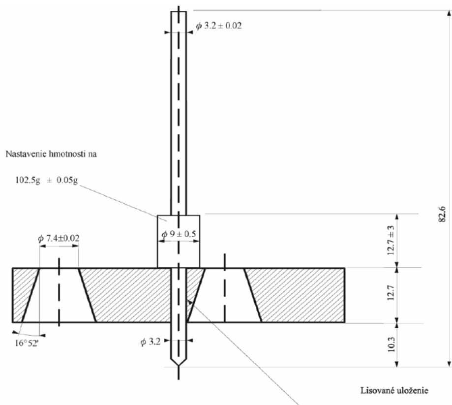
Obrázok 1 - Penetrometer
